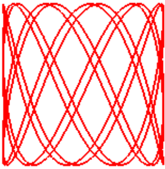
La courbe de Lissajous
